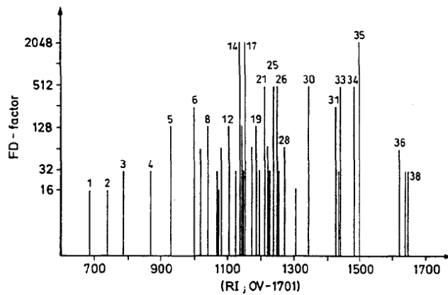
Şekil 5. Öğütülmüş ve kavruşmuş kahve aroma ekstraktının kromatogramı [31].
