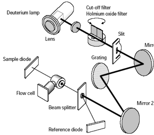
Şekil 6. Konvansiyonel değişebilir dalga boyu HPLC detektörü [37].
