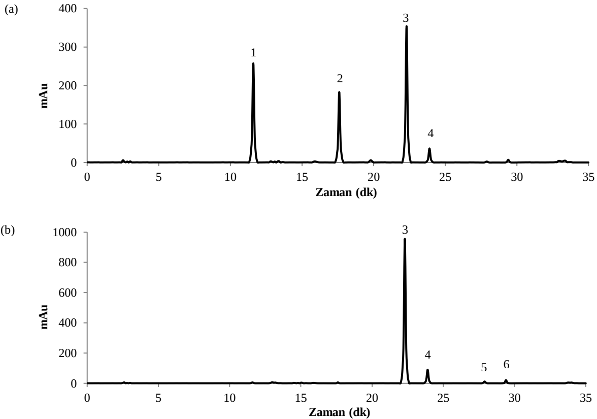
Şekil 1. İlaç formundaki Ginkgo biloba’nın asitsiz ekstraktının (a) 280 nm ve (b) 360 nm’deki HPLC kromatogramları (1:Protokatekuik asit, 2: p -hidroksi benzoik asit, 3:Rutin, 4:Kamferol-3-glikozit, 5:Kuersetin, 6:Kamferol)
