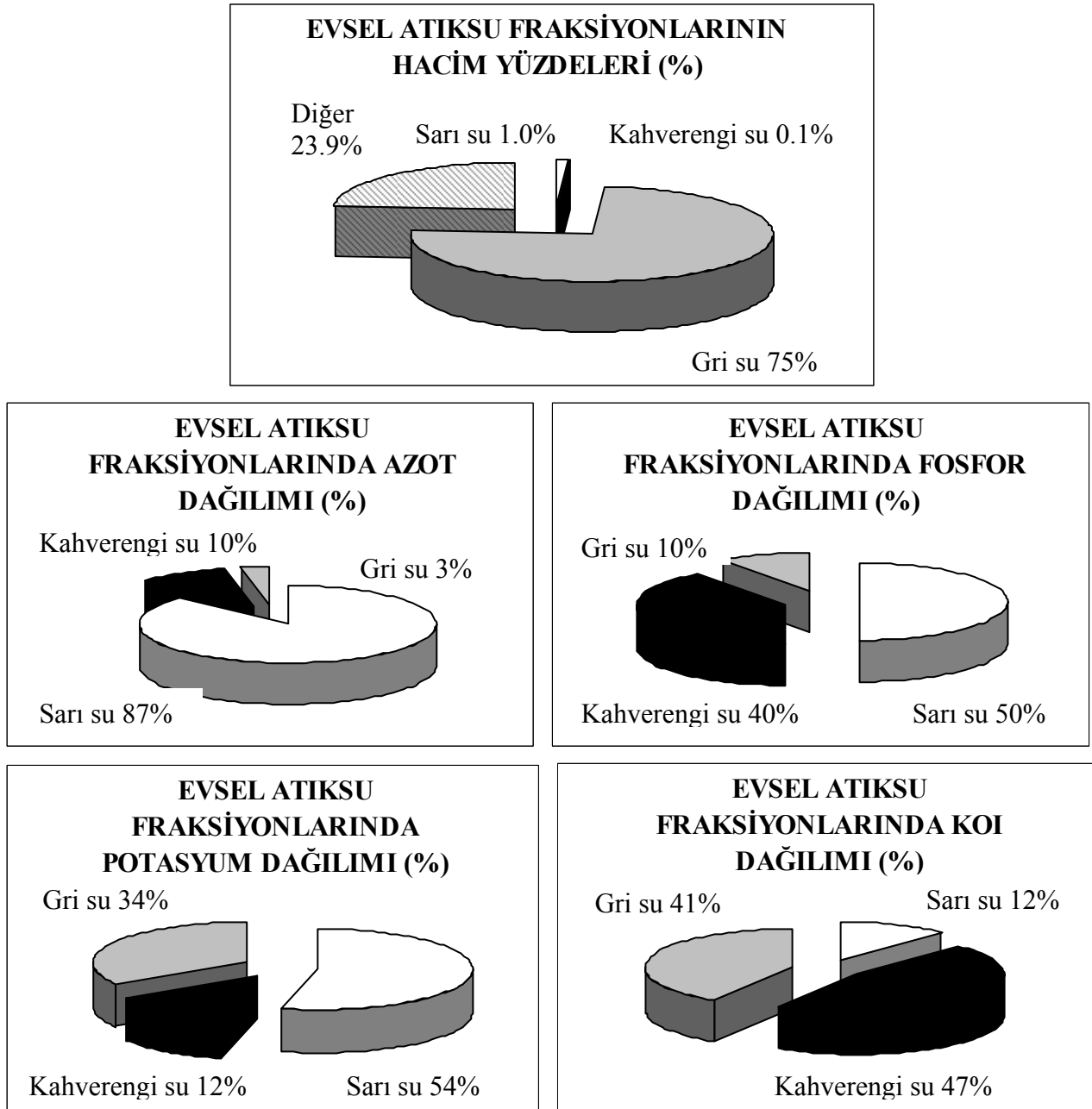
Şekil 2. Evsel atıksu bileşenleri (Belir Baykal, 2006)
