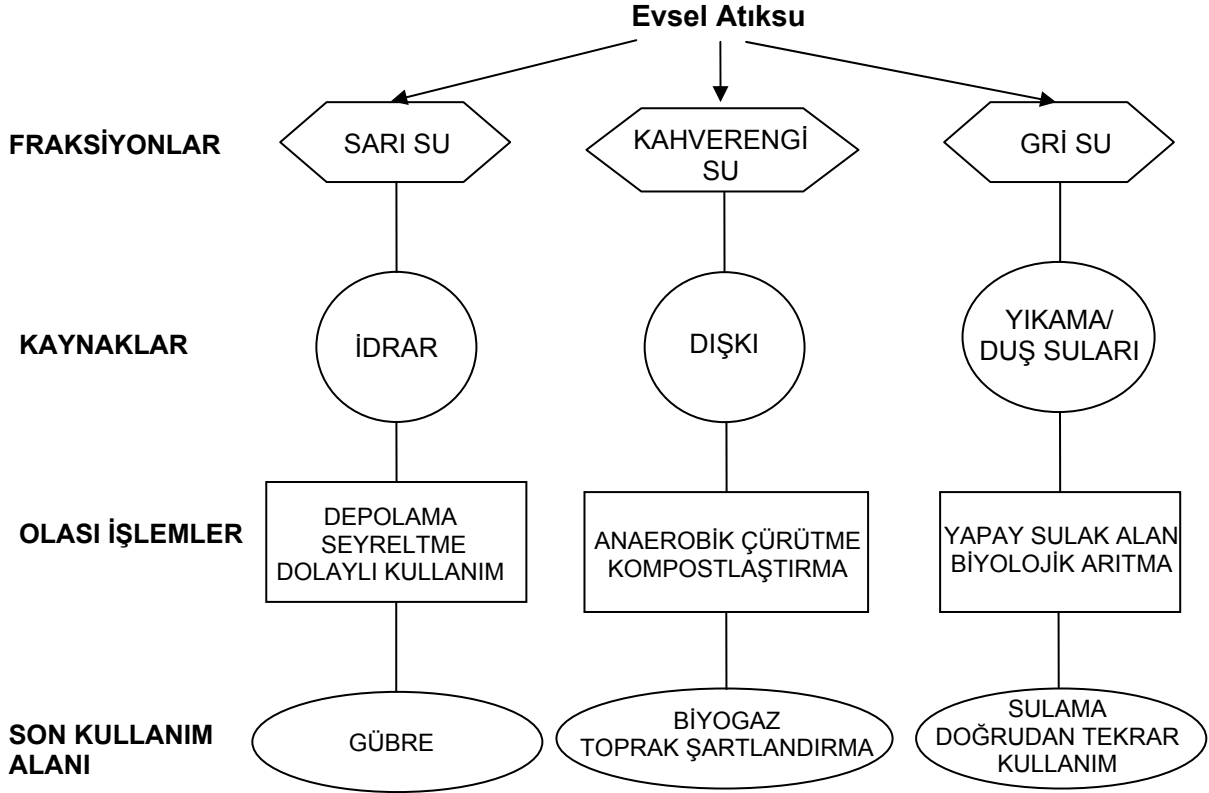
Şekil 3. Evsel atıksu fraksiyonları (Belér Baykal, 2006)
