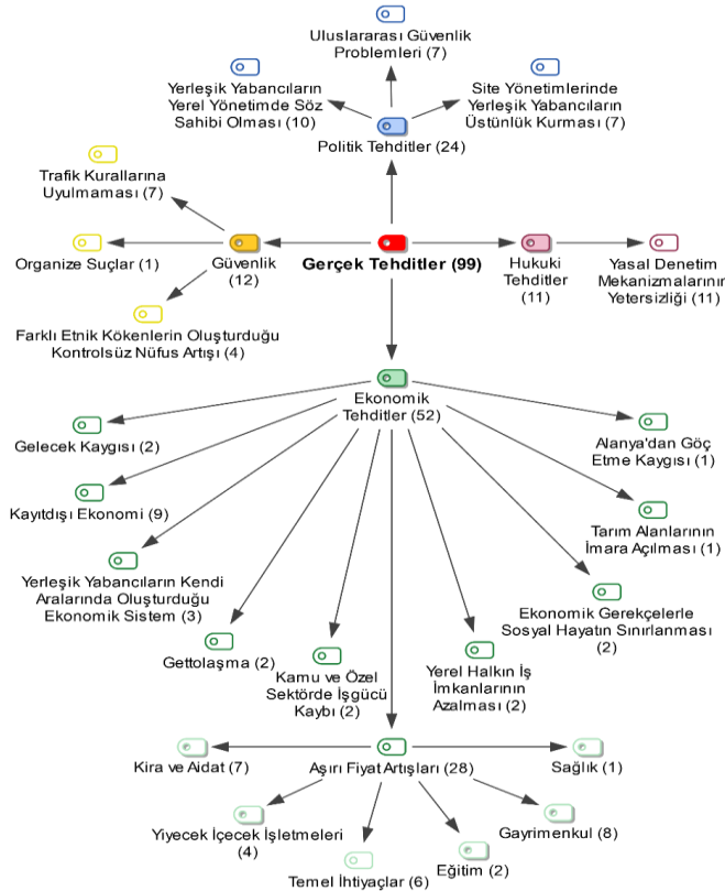
Şekil 1. Gerçek tehditler
