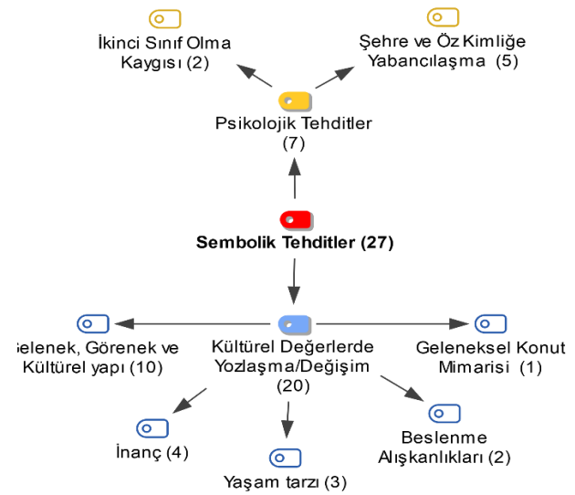
Şekil 2. Sembolik tehditler
