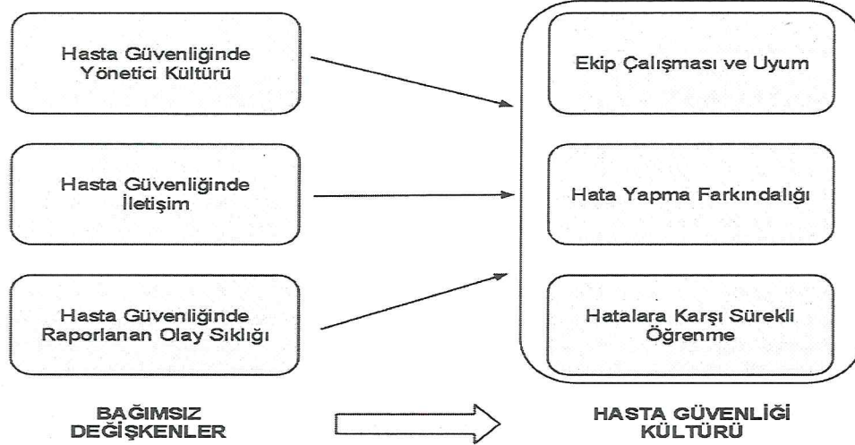
Şekil 1. Araştırmanın Modeli
