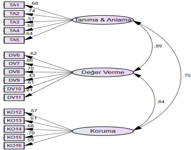
Şekil 3. KMDÖ'ye ilişkin DFA ve faktör yükleri
