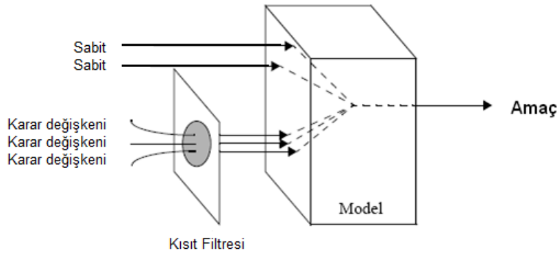
Şekil 1. Deterministik optimizasyon modeli [11]
